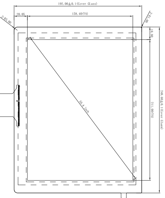
正视图
