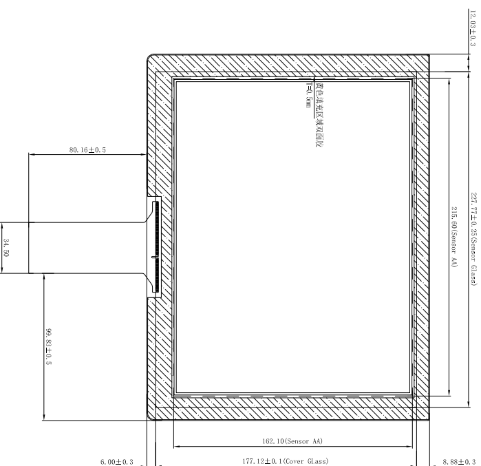
背视图
